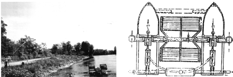
Slika 5. Sistem duo klipne pumpe POENIK u radu
