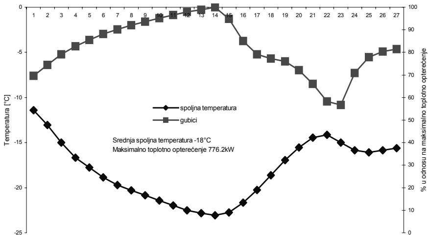
Slika 4. Profili opterećenja grejanja – srednja temperatura vazduha - 18 0 C
