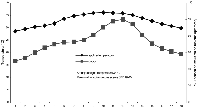
Slika 3. Profili opterećenja grejanja – srednja temperatura vazduha 33 0 C
