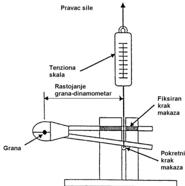
Slika 1. Šema postolja za testiranje
