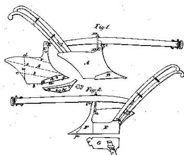
Sl. 7. Plug Džetro Vuda
