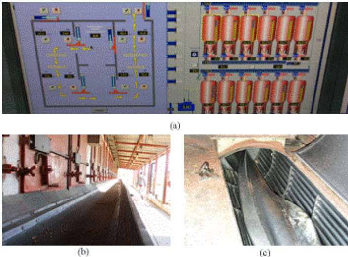
Slika. 3. Automatska regulacija Figure 3. Automatic regulation
