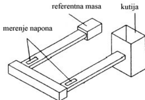
Slika 6. Uređaj za određivanje gustine
