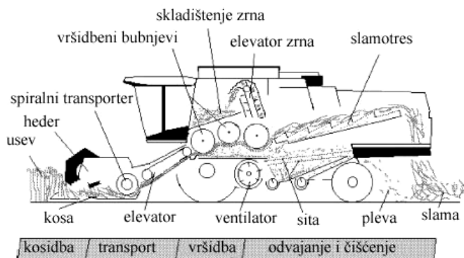
Slika 1. Proces koji se odvijaju na žitnom kombajnu sa klasičnom tehnološkom šemom
