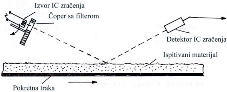
Slika 7. Prikaz rada infracrvenih merača vlažnosti čvrstih materijala, /5/
