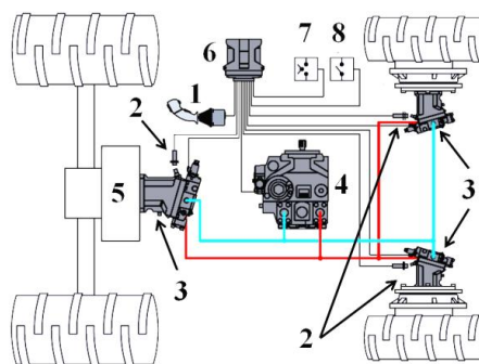
Slika 7. Hidrostatski pogon kombajna klipno-aksijalnim mašinama. [1]. Figure 7. Hydrostatic propulsion of harvester by piston-axial machines. [1].
