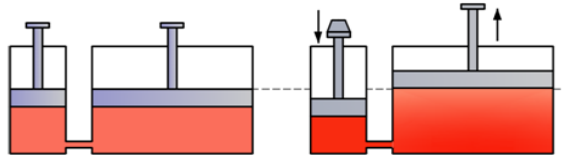
Slika. 1.1. Osnovni princip rada hidrostatičkog prenosnika - pojačavanje radne sile
