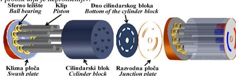
Slika 4. Klipno-aksijalna pumpa sa nagnutom kliznom pločom.
