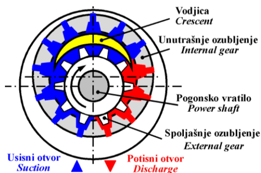
Slika 3. Zupčasta sa unutrašnjim ozubljenjem i vodicom (srpom).
