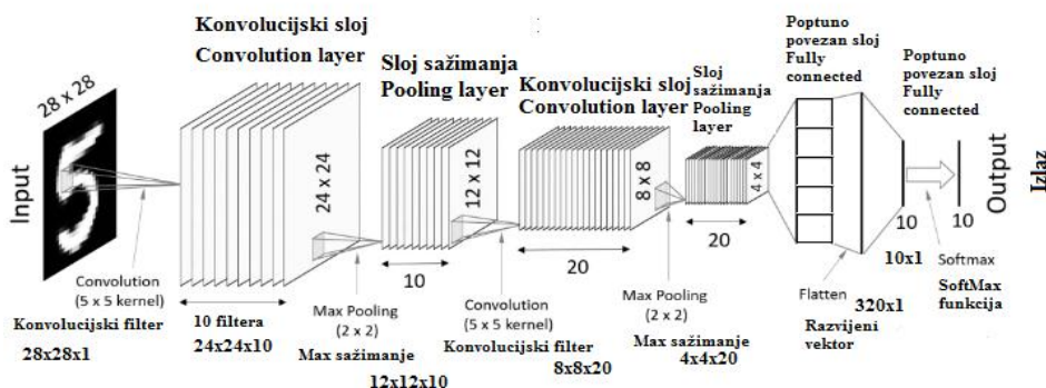
Slika 1. Primer arhitekture CNN mreže sa svim slojevima, [11].
