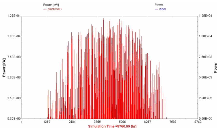
Slika 5. Časovne vrednosti toplote hlađenja u zoni gajenja, t_u=33^{\circ}\text{C} , \varphi=50\%
