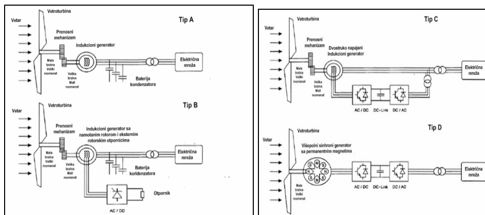
Slika 3. Tipične konfiguracije konverzionih sistema vetrogeneratora
