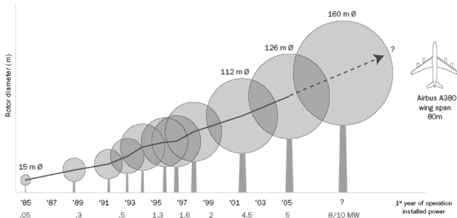
Slika 2. Porast instaliranih snaga i prečnika rotora vetroturbina
